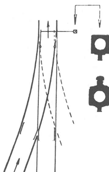
Mytävaihte on poikkeavalle raiteelle
