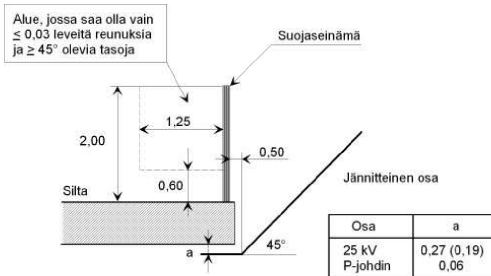
Kuva 5.9.16 Jännitteisten osien vähimmäisetäisyys suojaseinämän reunasta ja kiipeämisen vaikeuttaminen (mitat metreinä)
