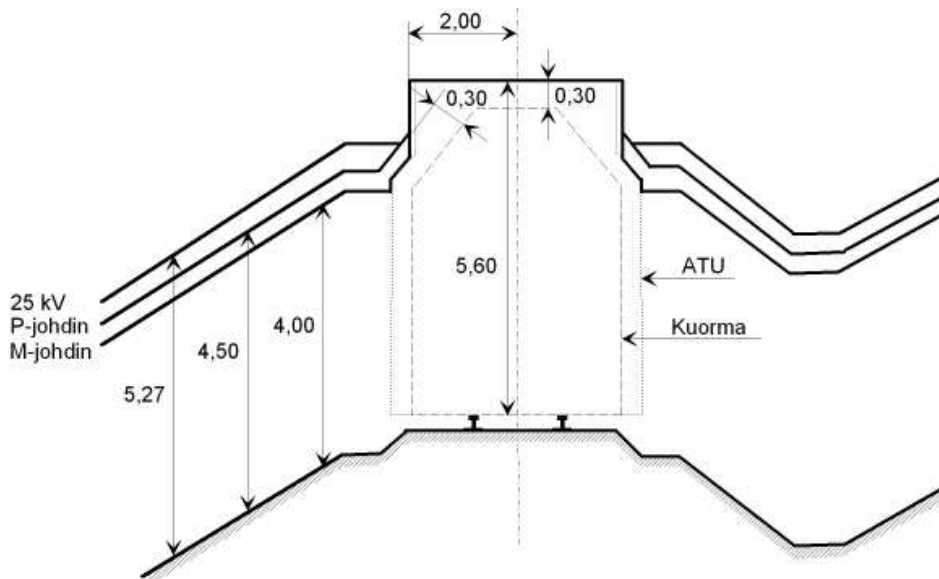
Kuva 5.9.1 Johtimien vähimmäisetäisyys avoradalla (mitat metreinä)
