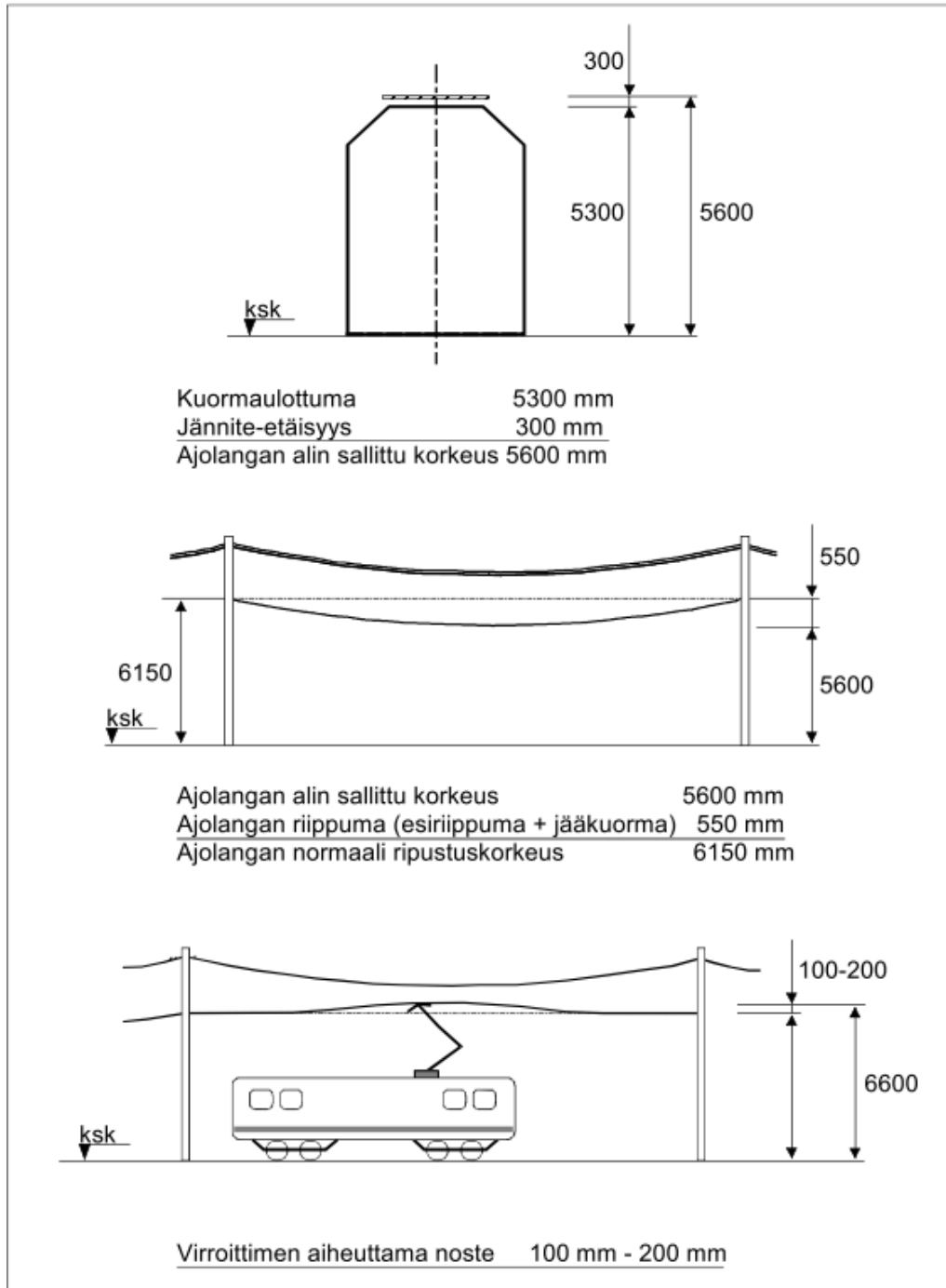
Kuva 5.6.3 Ajolangan korkeus
