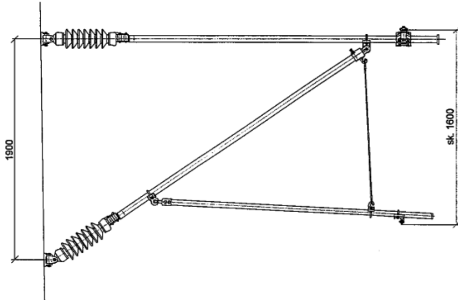
SIVURAITTEEN 2-ERISTIMINEN ORSI
