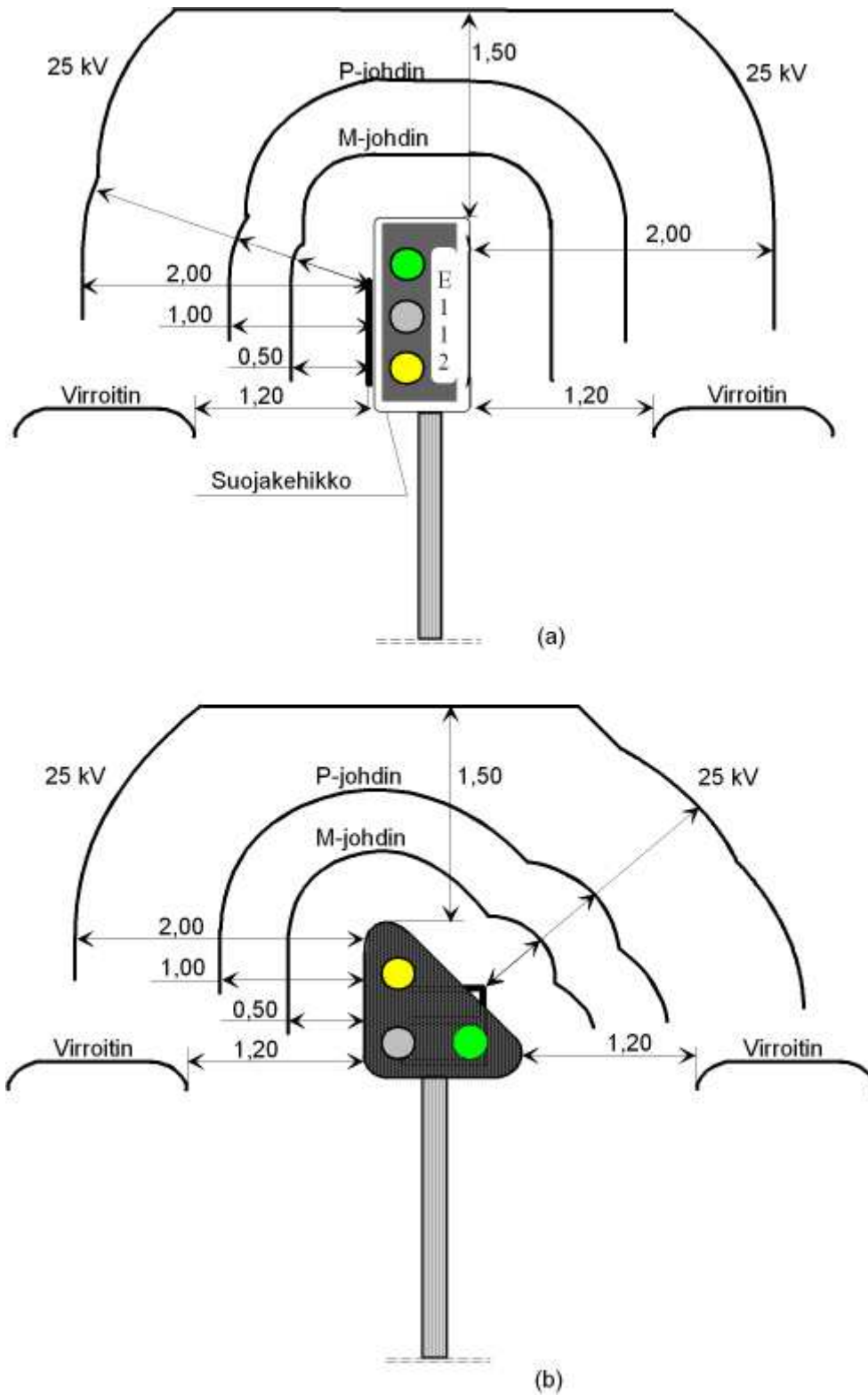
Kuva 5.9.10 Johtimien ja virroitinien vähimmäisetäisyydet opastimesta (mitat metreinä)
