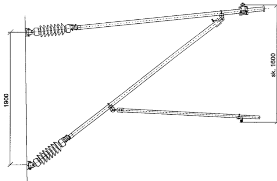
VÄLIPYLVÄÄN SIVUUNVIENTORSI
