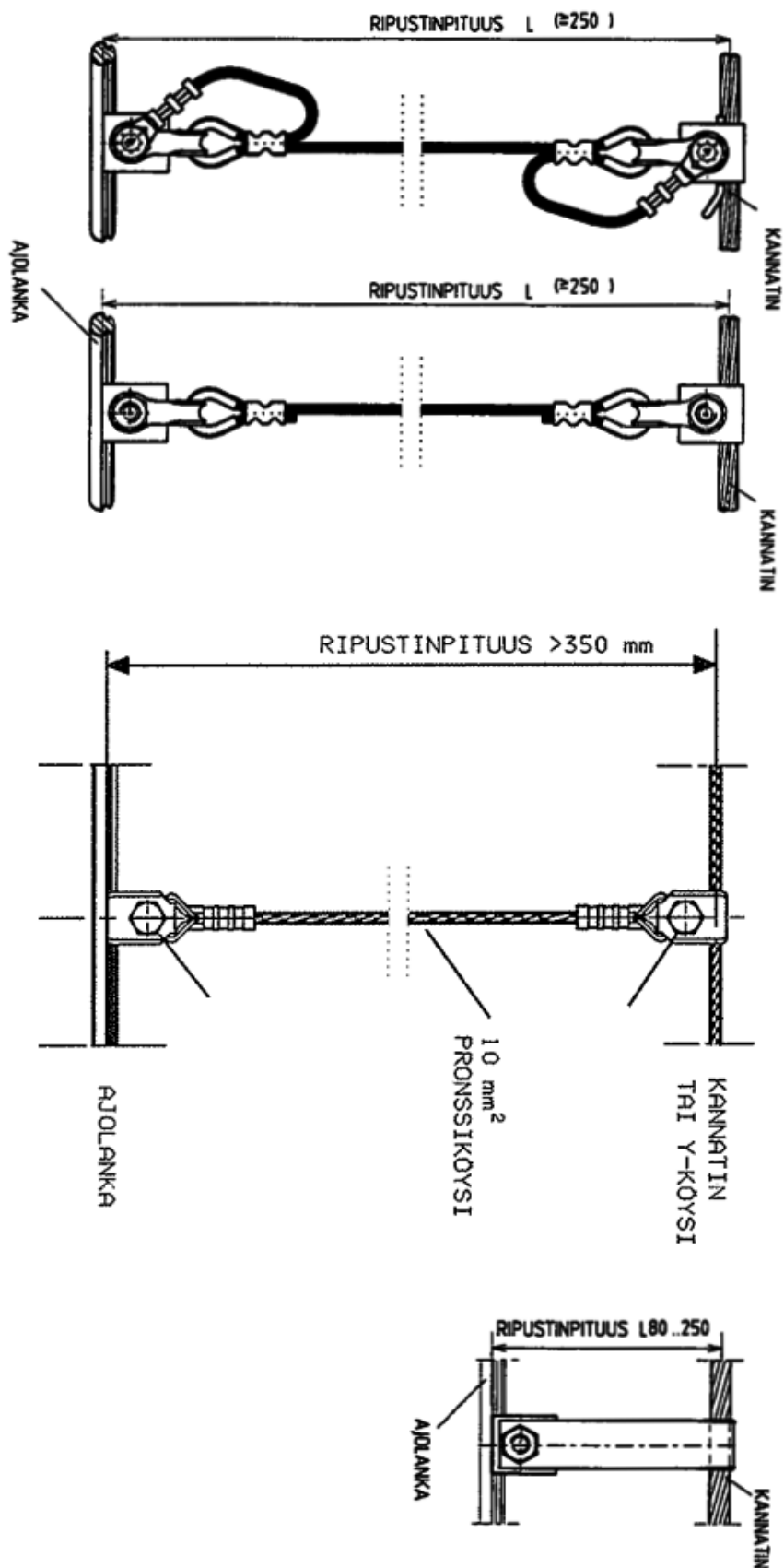
ERILAISIA RIPIUSTINTYYPPEJÄ
