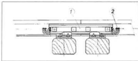
1 Sidekisko, 2 2 kpl johdinlenkkejä Kuva 11.7:6 Kiskon jatkoksen johdinlenkitys
