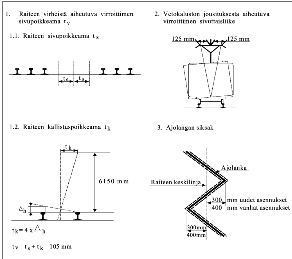
Kuva 5.6.2 Virroittimen yläosan sivuttaisliikkeen mitoitusperusteita ja ajolangan siksak
