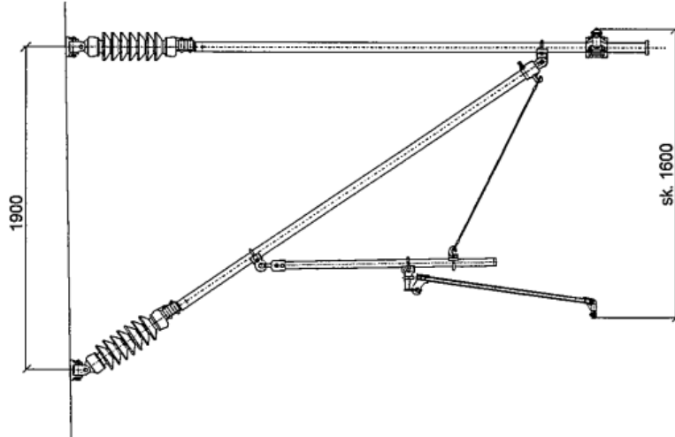
PÄÄRAITEEN VETO-ORSI
