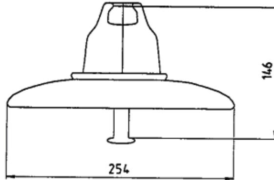
Laufaseristin
