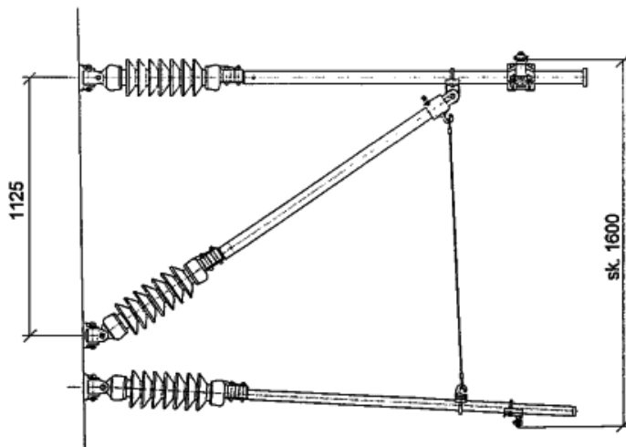
SIVURAITTEEN 3-ERISTIMINEN ORSI
