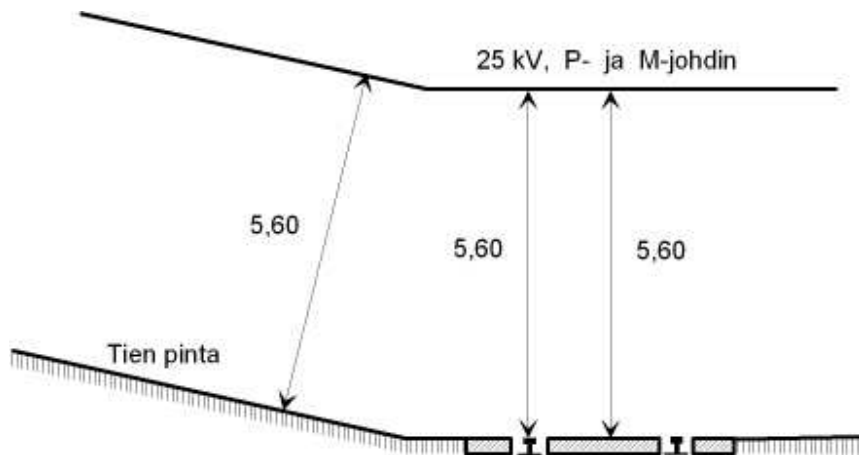
Kuva 5.9.2 Johtimien etäisyys kiskon selästä ja tien pinnasta tasoristeuksessa (mitat metreinä)
