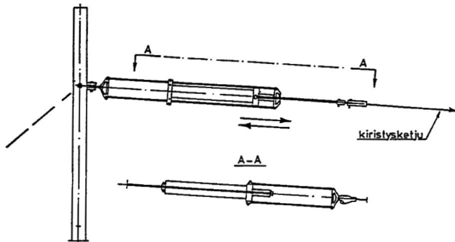
PNEUMAATTISHYDRAULINEN KIRISTYSLAITE
