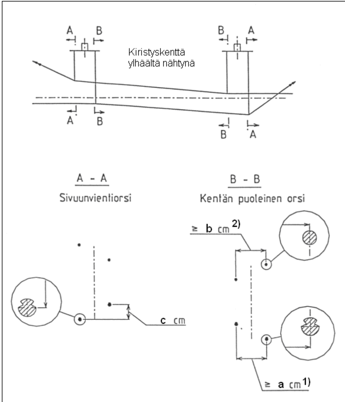
Kuva 5.7.2 Ajolankojen ja kannattimien keskinäinen asema kiristyskentän siirtymäjänteen ripustuskohdissa
