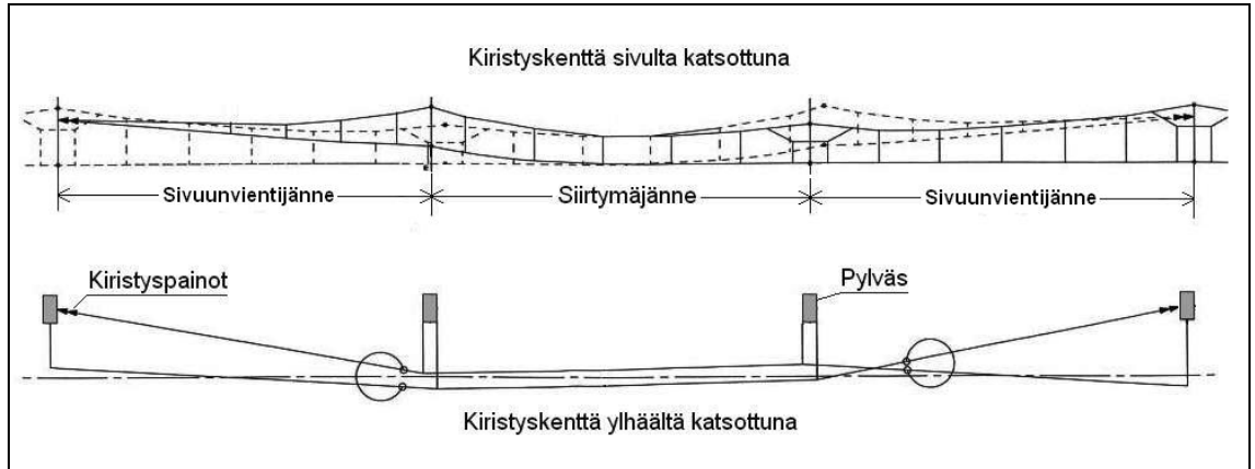
Kuva 5.7.1 Johtimien asettelu kiristyskentän siirtymäjännteessä; suljetussa kentässä yksi virtaliitântä ja erotuskentässä kaksi potentiaaliliitântää
