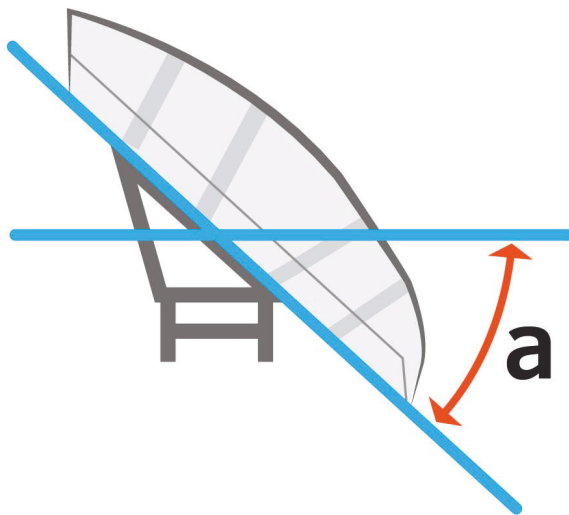
Kuva 22. Aurauskulma ( a ) on positiivinen oikealle aurattaessa.
