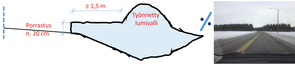
Kuva 35. Lumivallin madaltaminen päällystetyllä tieverkolla.
