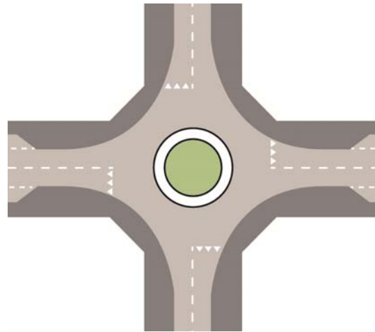
Kuva 106. Pyöräilyn sekaliikennetarkaisu kiertoliittymässä.
