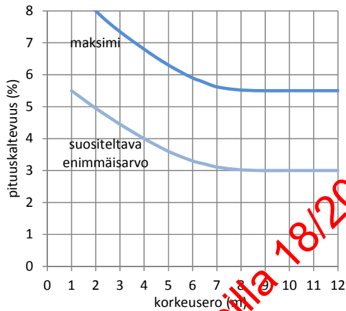
Kuva 63. Pituuskaltevuuksien mitoitusarvot korkeuseroon ja kaltevan matkan pituuteen verrattuna.
