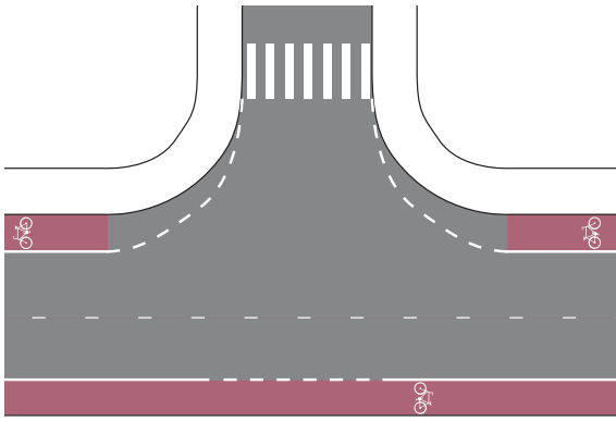
Kuva 156. Pyöräkaista tasa-arvoisessa risteyksessä.
