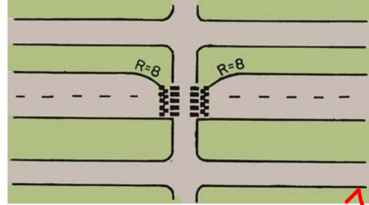
Kuva 105. Yksipuolinen kavennus risteäksen jalankulku- ja pyörätien kohdalla.
