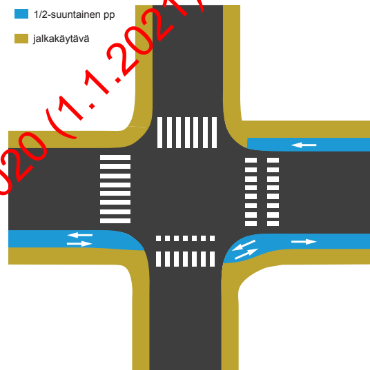
Kuva 45. Kaksisuuntainen pyörätie muuttuu risteyksen vaikutusalueella yksisuuntaiseksi pyörätieksi.
