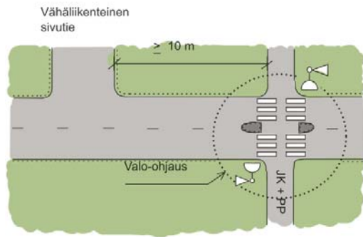
Kuva 110. Valo-ohjatun suojatien tai pyörätien jatkeen vähimmäisetäisyys valo-ohjaamattomasta kolmihaaraisesta risteyksestä (LVMa 1012/2001, 6 §).
