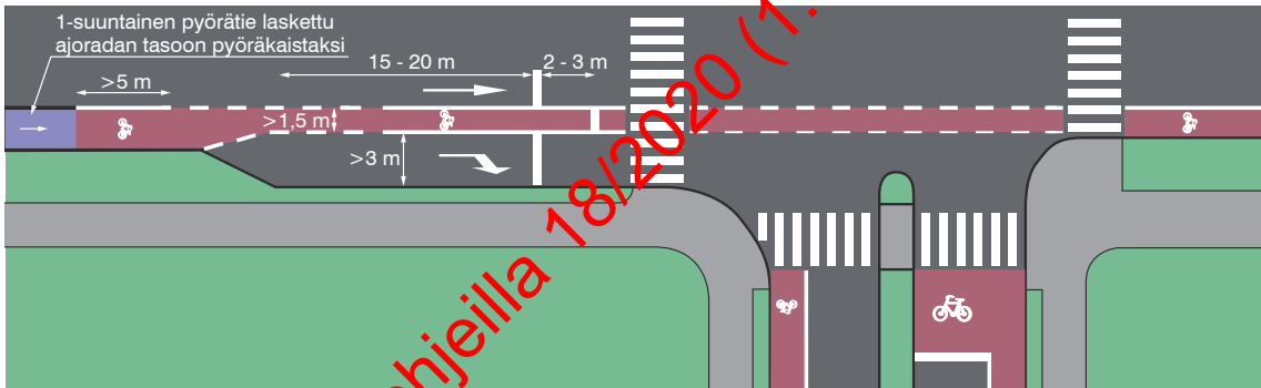
Kuva 42. Pyöräkaistan merkitseminen pääsuunnassa kääntymiskaistan kohdalla.
