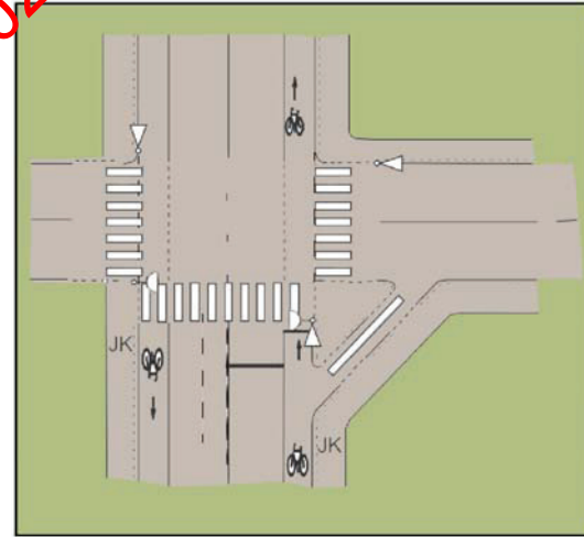
Kuva 119. "Vapaa oikea" pyöräilijöille. Järjestely voidaan tehdä myös pyöräkaistattoniin ratkaisuihin.
