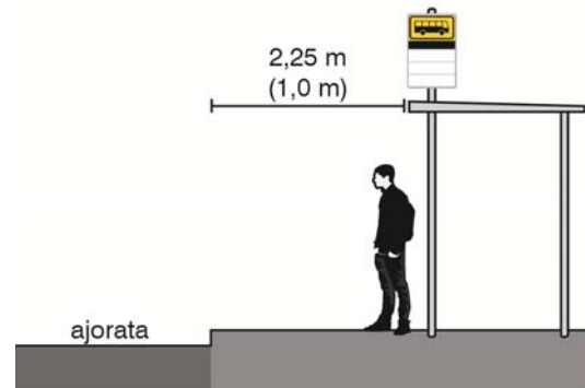
Kuva 53. Odotustilan mitoitus.
