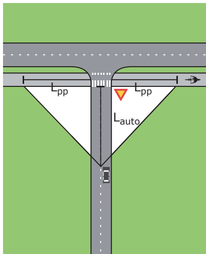
Kuva 73. Näkemäalueen määrittäminen tasoliittymän yhteydessä olevassa pyörätien sekä ajoradan risteyksessä, kun autoliikenne on väistämismittainen. Pyöräiliikenteen ollessa väistämismittainen sovelletaan kuvan 72 mukaisia L auto -arvoja.
