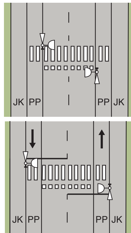
Kuva 112. Esimerkki ajoradan suuntaisesta ajoradalla kiinni olevasta valo-ohjatusta ja valo-ohjaamattomasta pyörätiestä.
