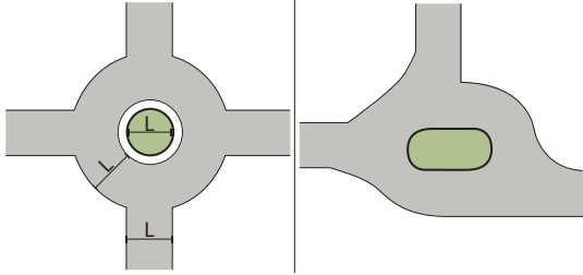
Kuva 123. Esimerkkejä pyöräilyn pääreittien risteyskohtien järjestelystä.
