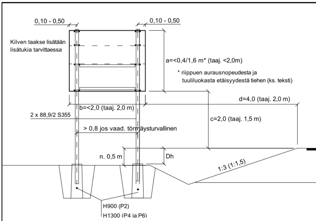
Kuva 20. Opastusmerkki kahdella 90/2 pylväällä, joka täyttää törmäysturvallisuusvaatimukset, kun kilven pinta-ala on <math>< 4,9 \text{ m}^2</math> ja alareunan korkeus vähintään 2,0 m ja kilpi irtoaa kiinnityksestään törmäyksessä eikä vaakatukia kiinnitetä pylväisiin.
