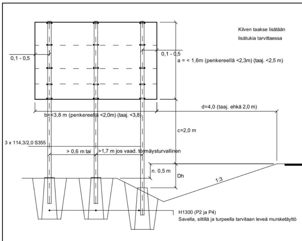
Kuva 24. Opastusmerkki kolmella tai useammalla 114/2 pylvällä. Ratkaisu ei ole törmäysturvallinen, jos pylväsväli on < 1,7 m k/k.
