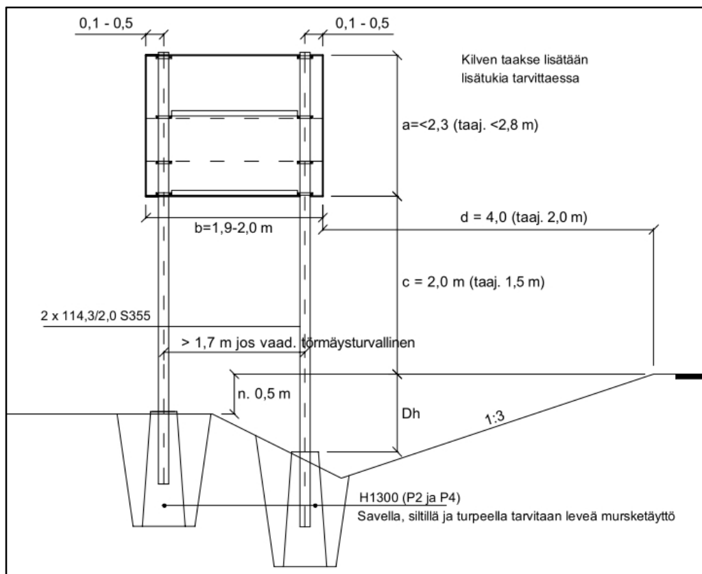
Kuva 23. Opastusmerkki kahdella 114/2 pylvällä täyttää törmäysturvallisuuden vaatimukset, kun kilven pinta-ala on < 4,0 m 2 ja kilven korkeus tiestä 2,0 m ja kun kilpi irtoaa kiinnityksestään törmäyksessä eikä vaakatukia kiinnitetä pylväisiin.
