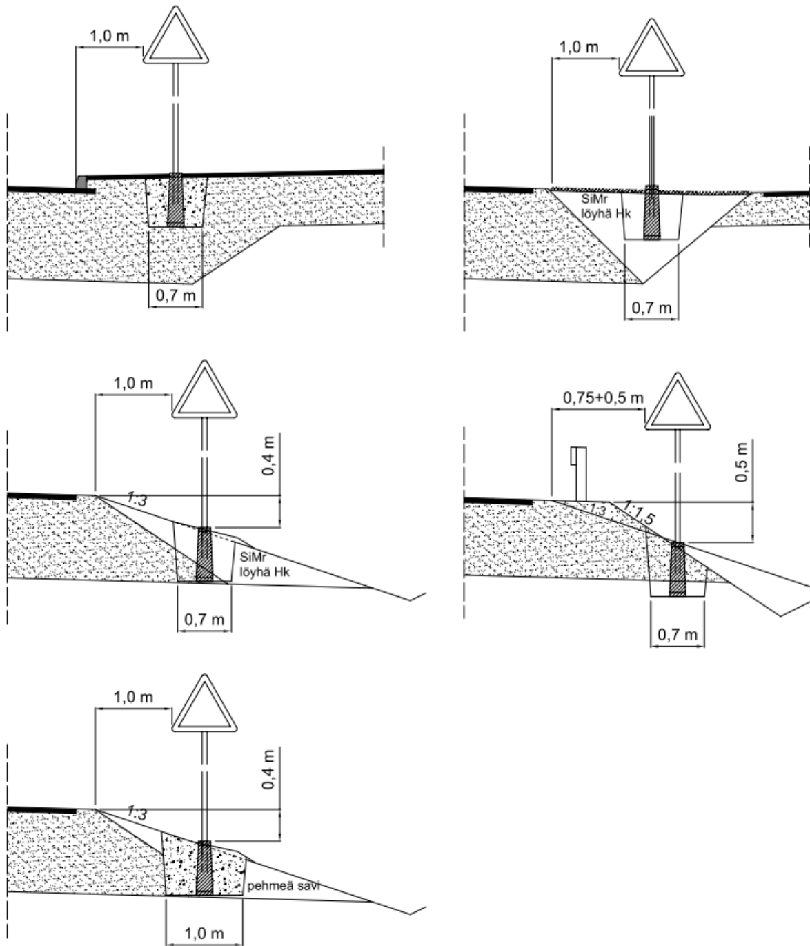
Kuva 1. Liikennemerkkin ja pylväsperustusten sijoittaminen eri luiskatilanteissa, sijoituksesta tarkemmin ohjeessa "Yleisohjeet liikennemerkkien käytöstä" Tieh 2000006-03.
