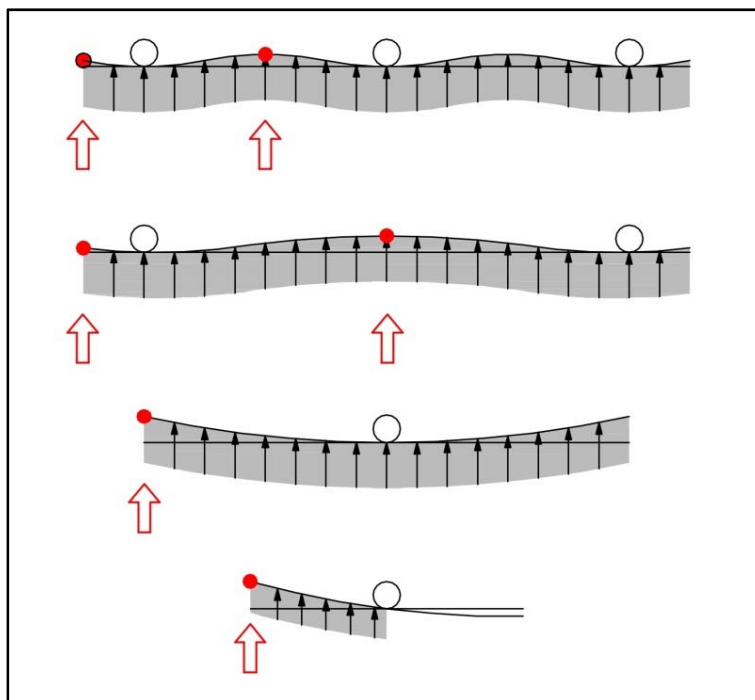
Kuva 1. Pohjamateriaalin reunan siirtymä tuulikuorman aiheuttaman taipuman vaikutuksesta todetaan nuolten ja punaisten pisteiden kohdalta, ja jaetaan havaintopisteen ja tukipisteen välimatkalla. Saaduista taipuma-arvoista valitaan suurin ja sitä verrataan sallittavaan taipumaan.
