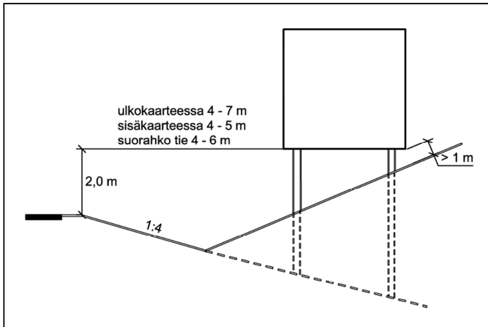
Kuva 14. Opastusmerkin sijoittaminen valta- ja kantateillä sekä kolmi- tai useampikaistaisilla teillä ja mahdollisuuksien mukaan muillakin maanteilla.
